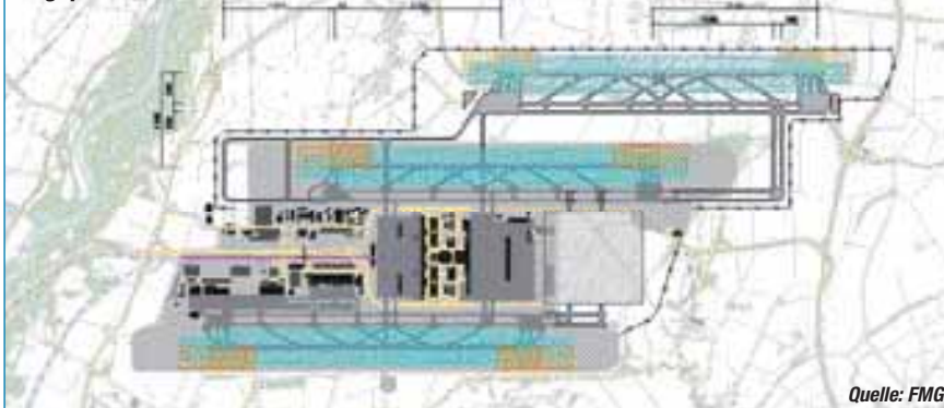
Lageplan der 3. Startbahn – Variante Vb
